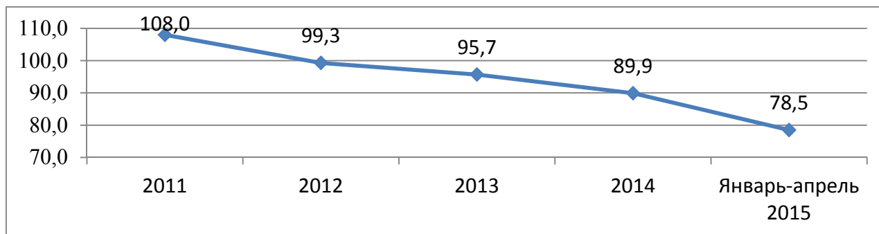
Рис. 1. Динамика индекса промышленной продукции в Украине
